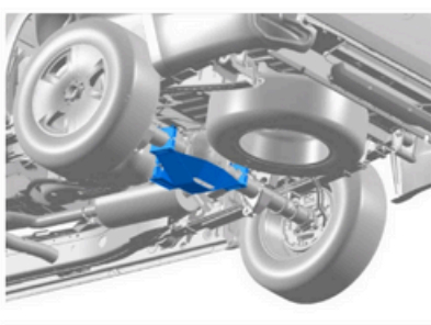
Protección y Conservación Protección diferencial - VW Amarok
